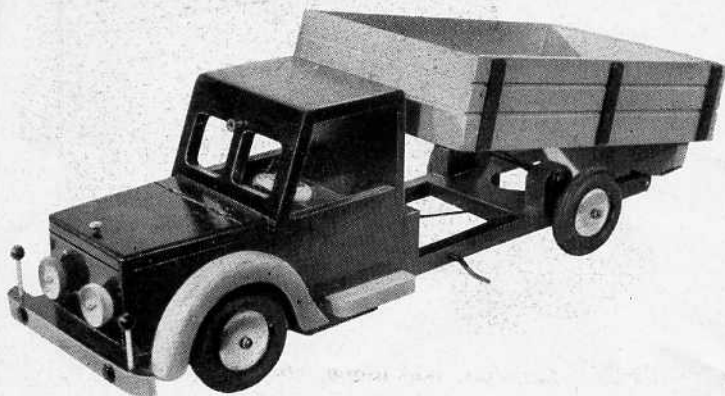
5270 — Camion bois laqué, éclairage électrique, interrupteur sur le volant, benne basculante avec manivelle de manœuvre, roues métal et pneus caoutchouc. Longueur 60 \frac{c}{m} . . . . . Pièce
